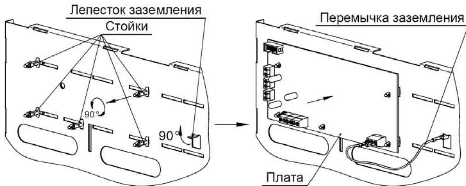
Рисунок 2: Установка платы.
