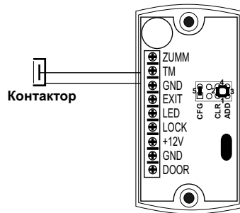
Рис.6 Подключение контактора
