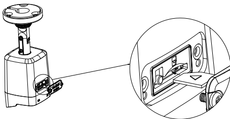
Рисунок 2-1 Демонтаж крышки и установка карты памяти
