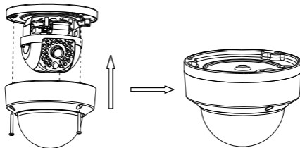
Рисунок 2-3-6 Установка купола
