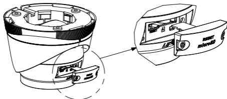
Рисунок 2-1. Снятие крышки и установка карты памяти
