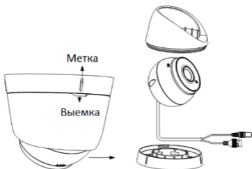
Рисунок 2-4-2 Демонтаж камеры
