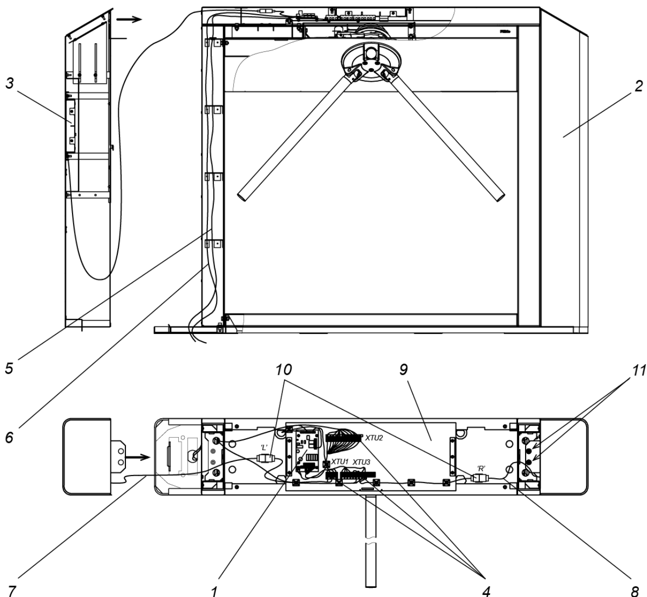
Рисунок 15. Схема прокладки кабелей в стойке турникета
