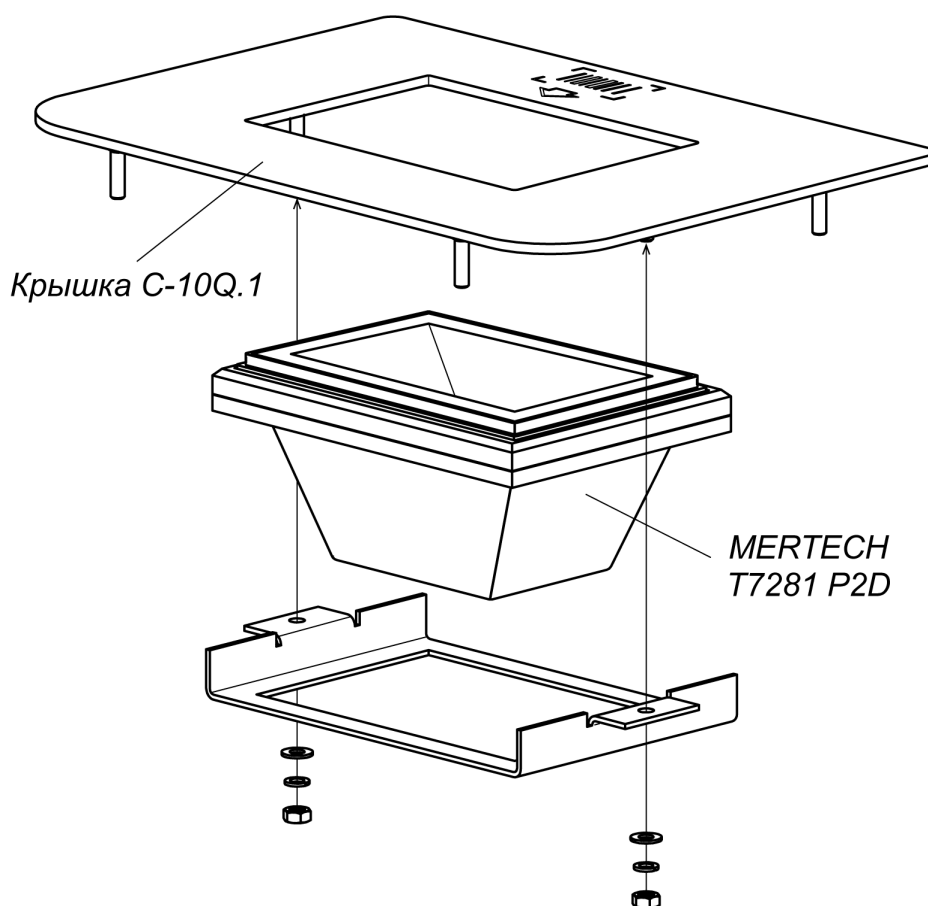
Рисунок 31. Боковая крышка PERCo-C-10Q.1 со сканером штрихкода Mertech T7281 P2D
