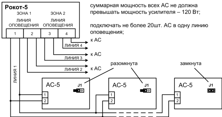
Рис.5б Схема подключений АС-5 к линиям оповещения
