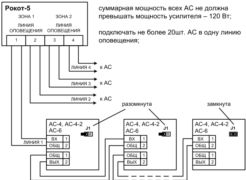
Рис.5а Схема подключений АС-4, АС-4-2, АС-6 к линиям оповещения
