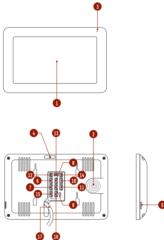
Рис. 2 Описание монитора видеодомофона FREEDOM 7 FHD (WIFI)
