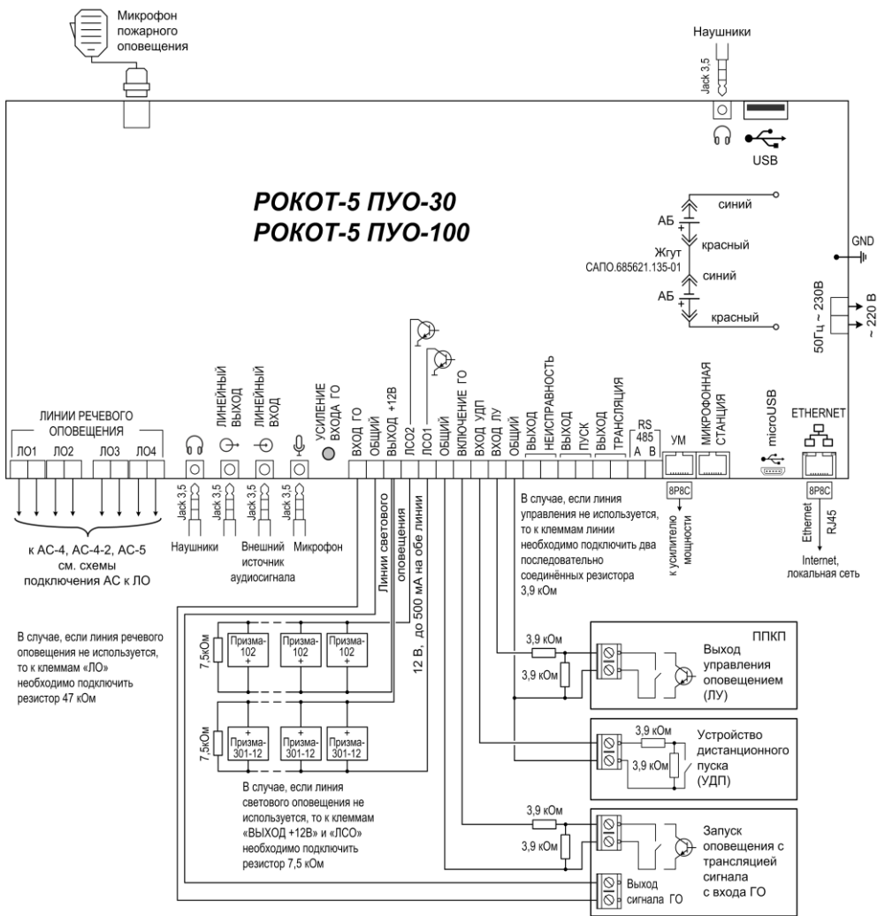
Рис.А1 Схема внешних подключений «РОКОТ-5 ПУО» (интерфейс RS-485 в данной версии ПУО не используется)
