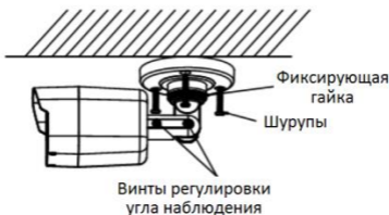
Рисунок 2-2 Установка камеры на потолок
