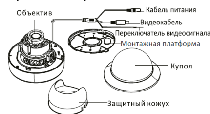
Рисунок 1-12 Купольная камера II типа
