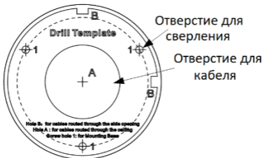
Рисунок 2.9 Шаблон крепления
