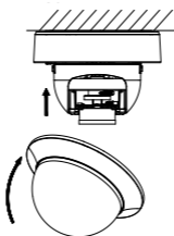
Рисунок 2.16 Завершение установки
