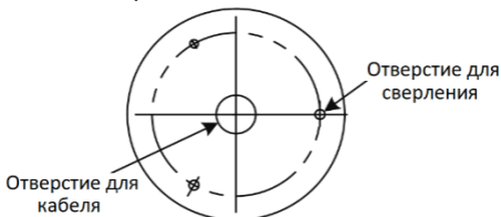
Рисунок 2.5 Шаблон крепления
