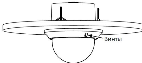
Рисунок 1-13 Установка купола
