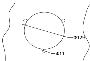
Рисунок 1-9 Шаблон крепления
