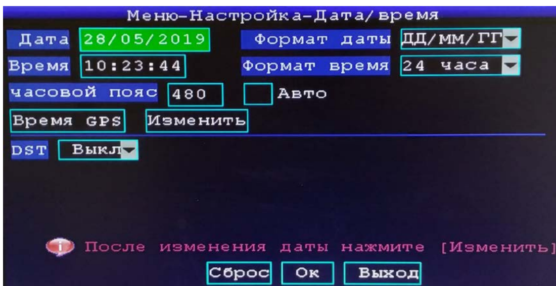
Рис.6 Настройки времени
