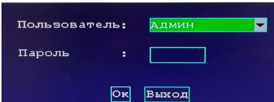
Рис.2 Авторизация
