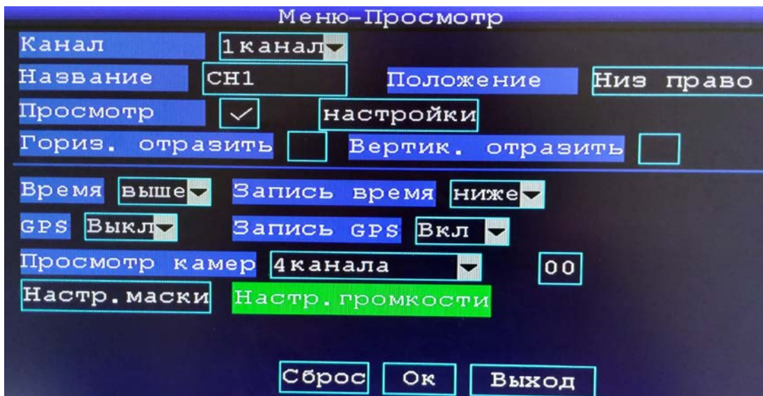
Рис.12 Настройки просмотра
