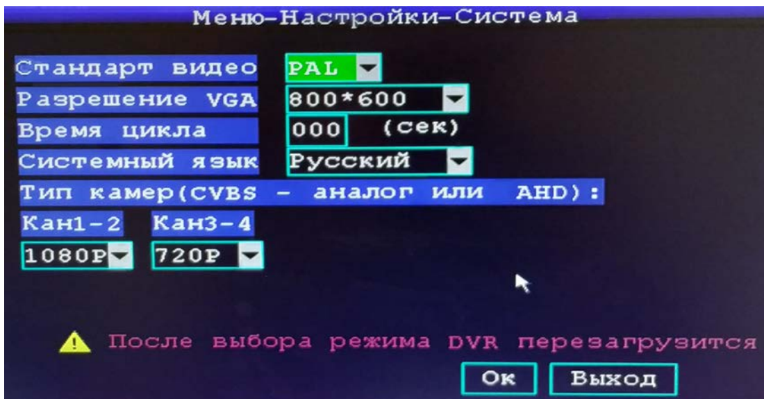
Рис.5 Настройки системы
