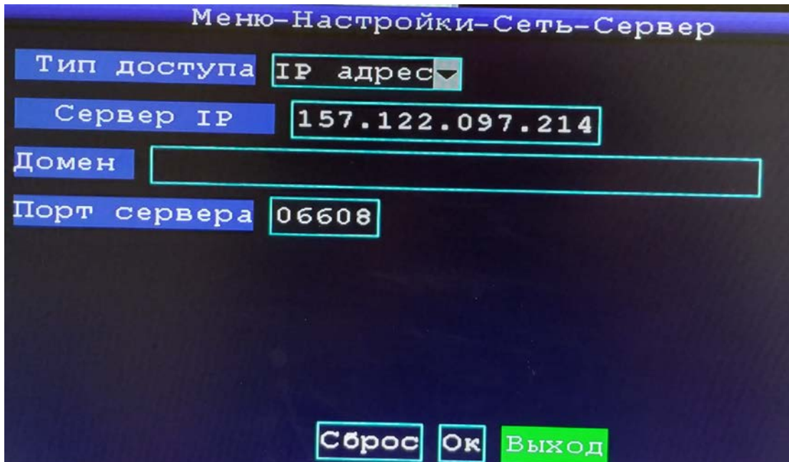
Рис.20 Настройка CMS
