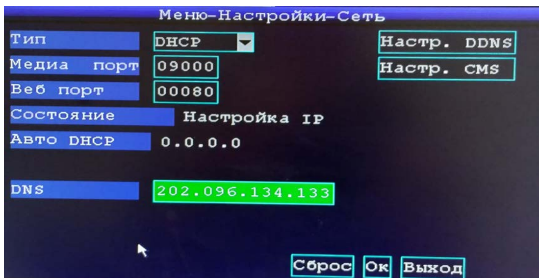
Рис.19 Настройка сети
