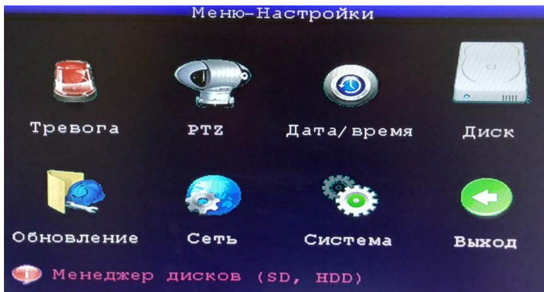
Рис.4 Настройки
