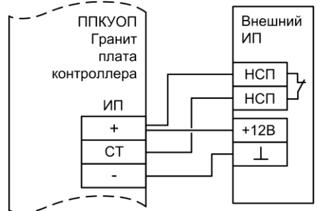
Рис.Б6 Схема подключения внешнего источника электропитания (ИП)
