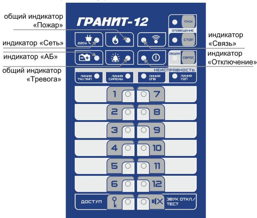
Рис.2 Панель индикации и управления прибора Гранит-12
