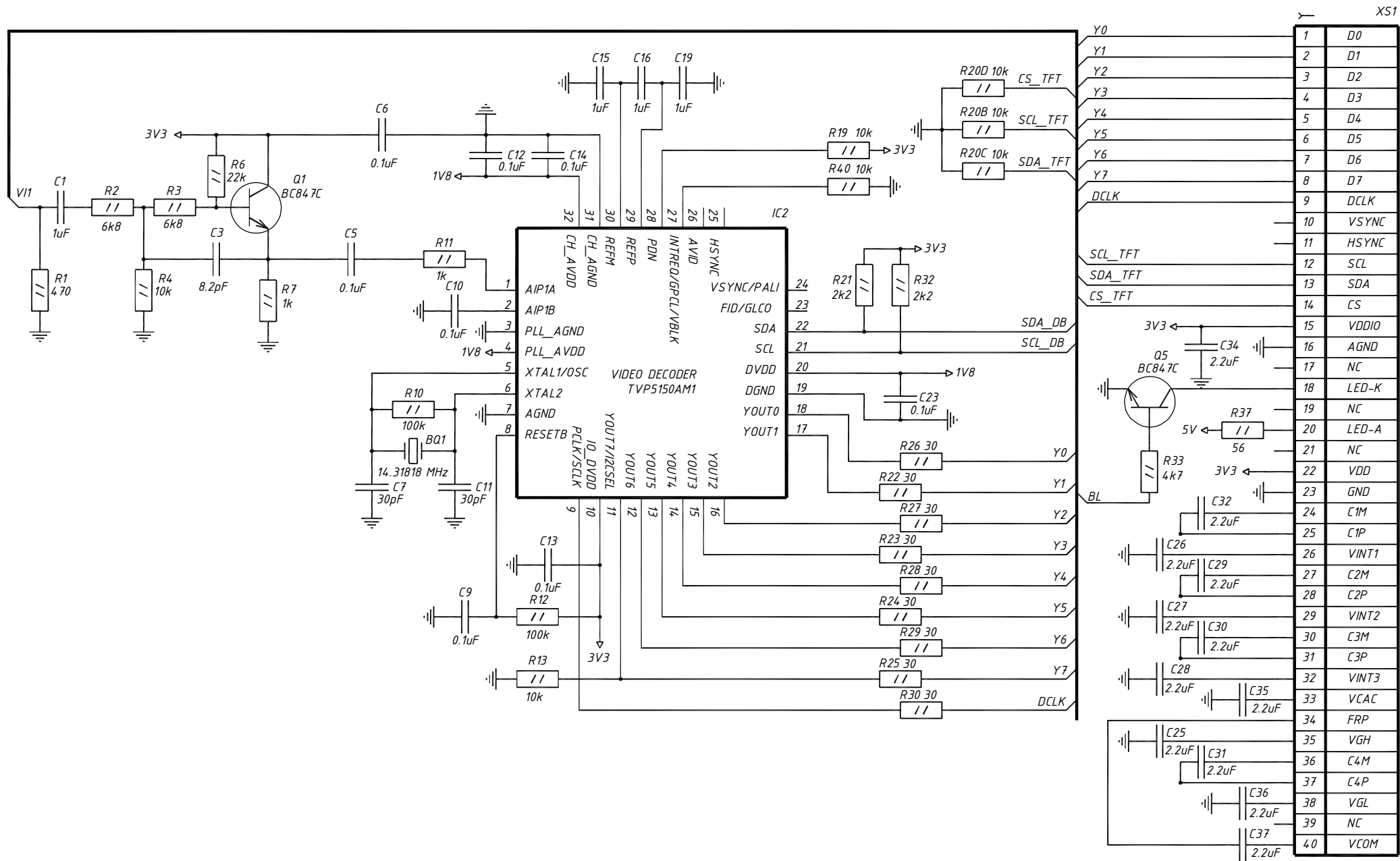
Модуль управления MU-327 Схема электрическая принципиальная
