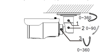
Рисунок 1-8 Настройка угла наблюдения камеры
