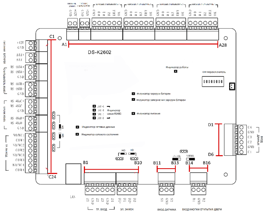
Рисунок 3-2 Описание клемм DS-K2602
