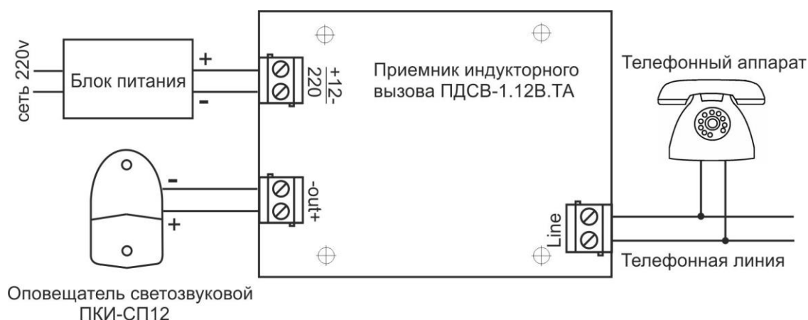
Рис.1 Схема подключения GC-0001C2
