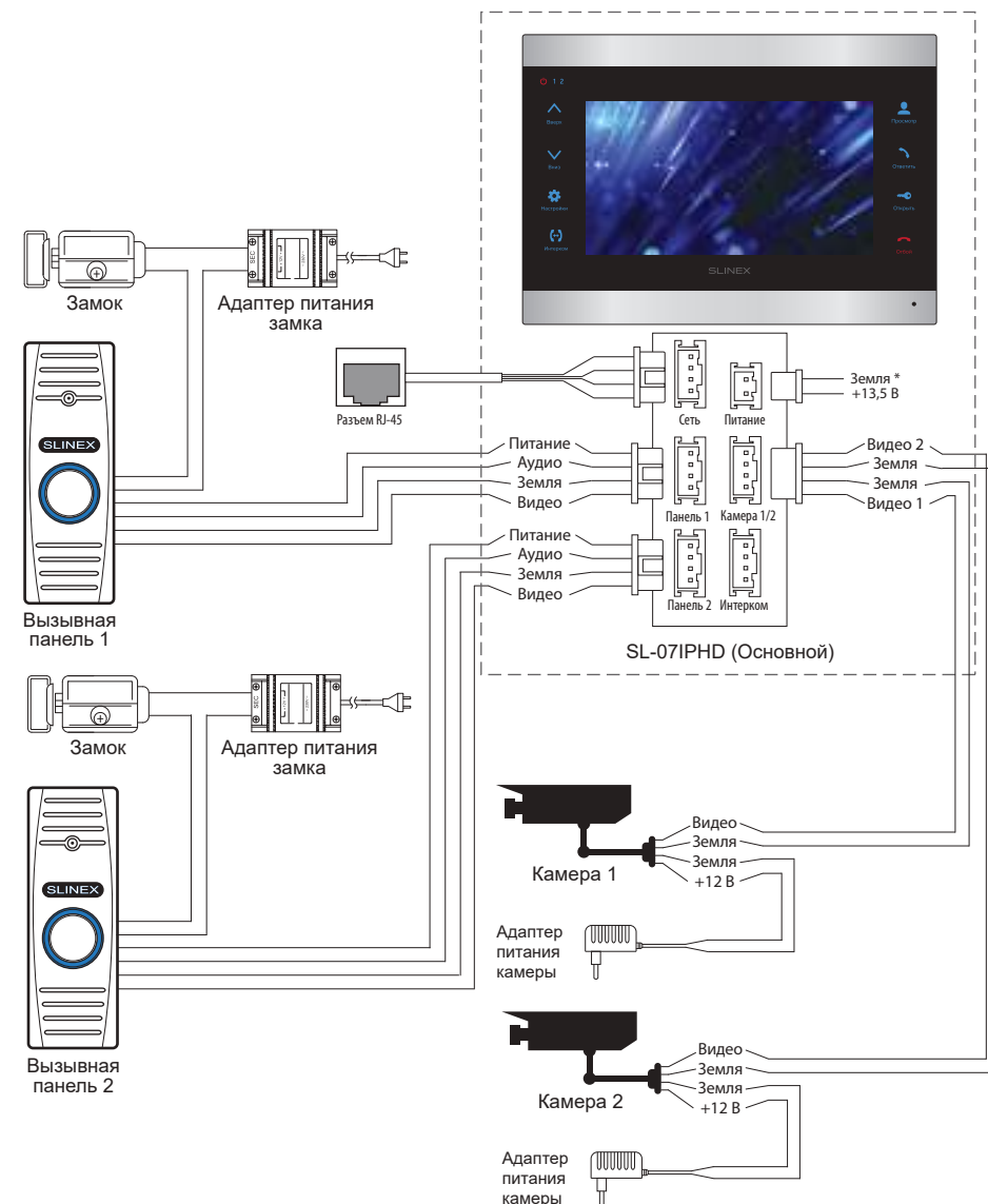
Схема 1. Подключение вызывных панелей и камер к домофону SL-07IPHD.
