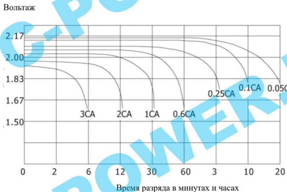
График Напряжение-остаточная ёмкость
