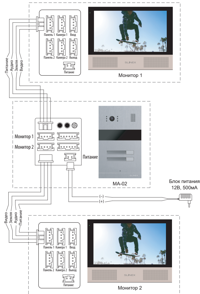
Схема 1. Подключение МА-02 с двумя мониторами.
