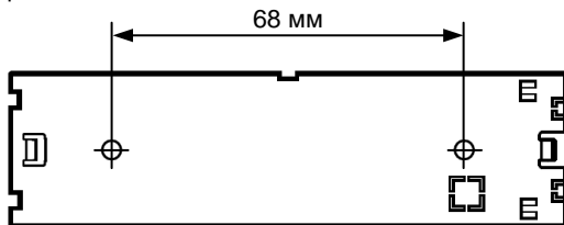
Рис.9 Присоединительные размеры
