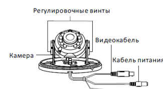
Рисунок 1-10 Купольная камера I типа
