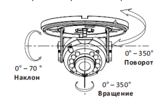
Рисунок 1-12 Настройка угла наблюдения камеры
