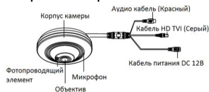
Рисунок 1-28 Панорамная камера
