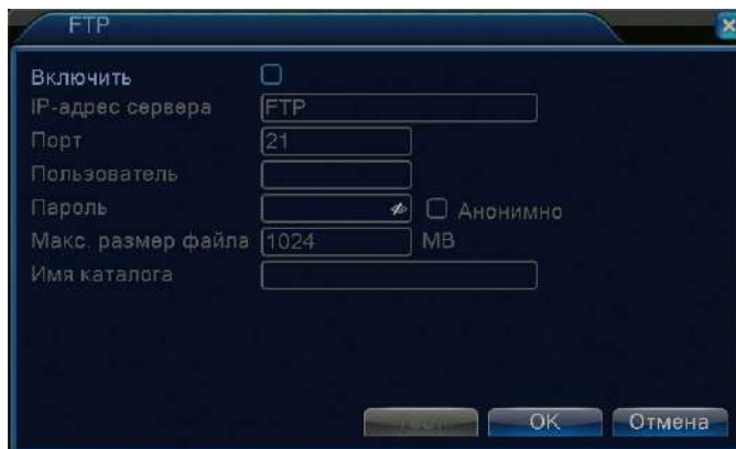
Рисунок 4.22 Настройки FTP
