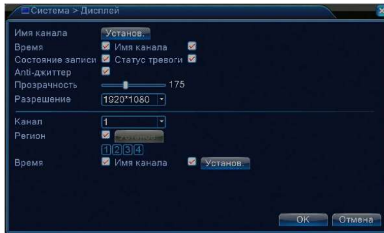
Рисунок 4.31 Включение маскирования
