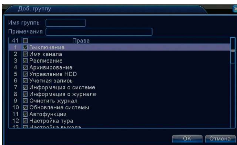
Рисунок 4.48 Добавить группу
