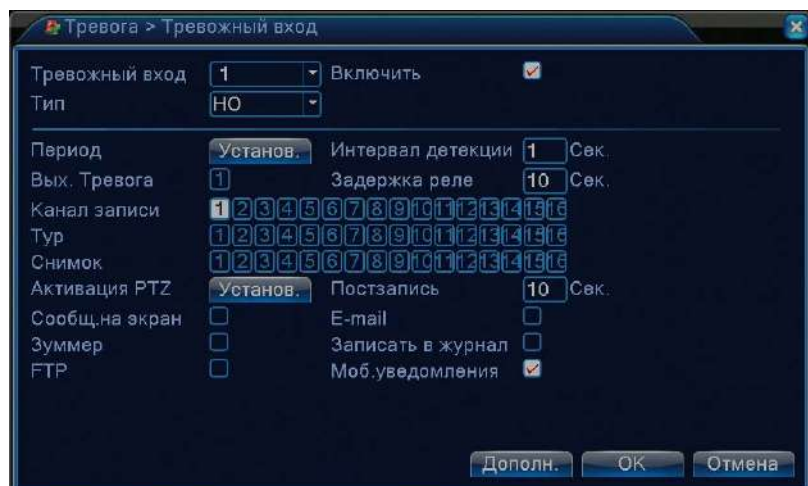
Рисунок 4.10 Вход Тревоги
