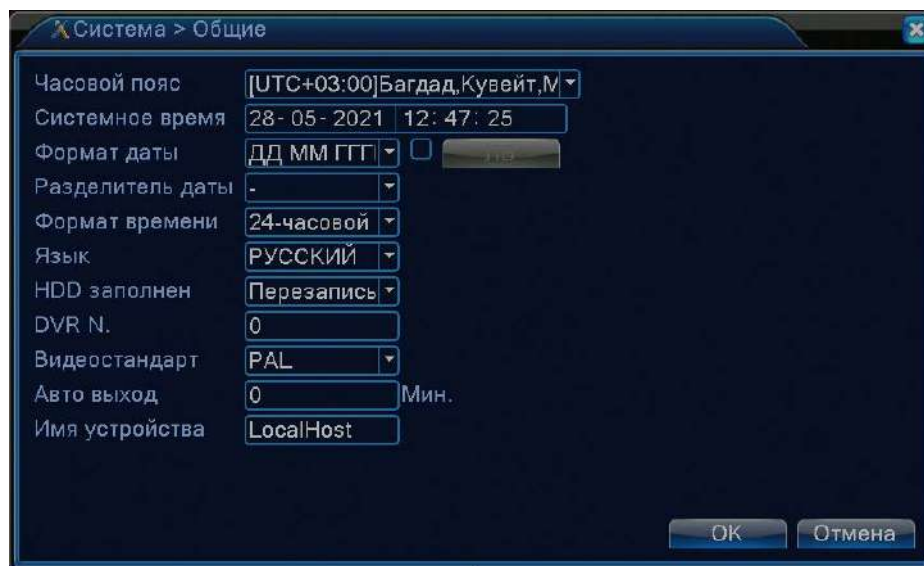
Рисунок 4.12 Общие настройки
