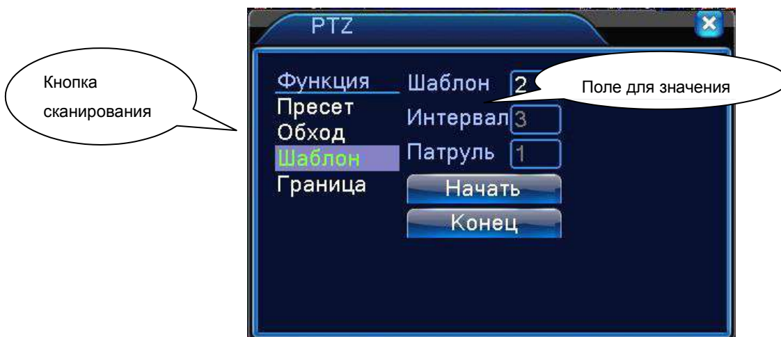
Рисунок 3.14 Настройки сканирования
