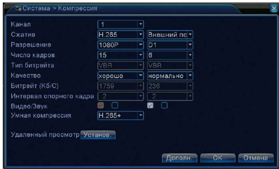
Рисунок 4.15 Настройки компрессии
