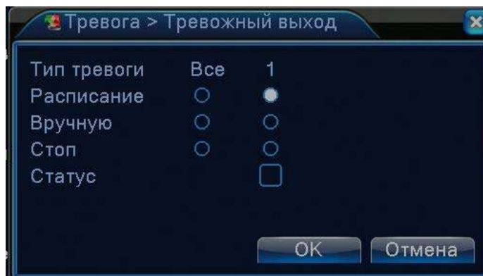
Рисунок 3.9 Тревожный выход
