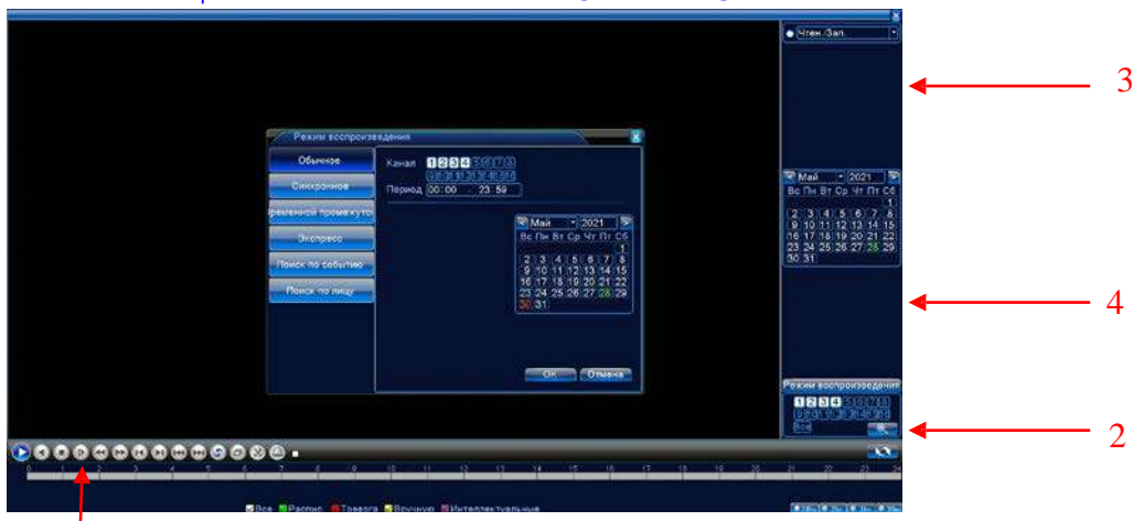
Рисунок 3.4 Воспроизведение видео
