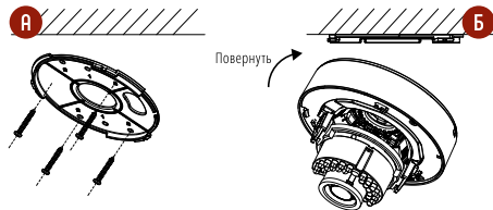
Рис. 6 Установка видеокамеры Н1Т ×6
