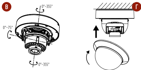
Рис. 7 Установка видеокамеры НIT x6
