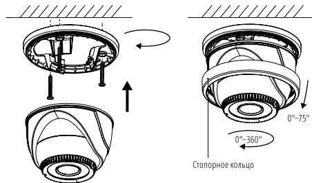
Рис. 8 Установка видеокамеры НIT x7
