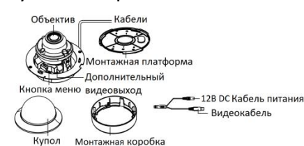
Рисунок 1-14 Купольная камера III типа
