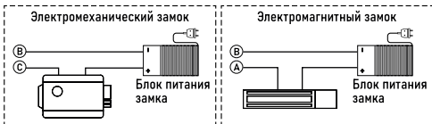
Схема подключения вызывной панели FANTASY MR/IRMK
