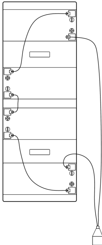
Рисунок 10 — схема соединений АКБ
