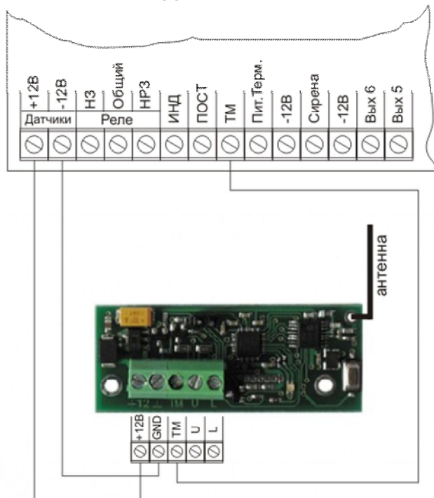
Клемная колодка Часовой 8x8-ВОХ
