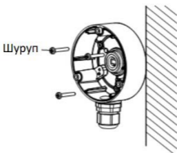
Рисунок 2-4 Установка монтажной коробки
