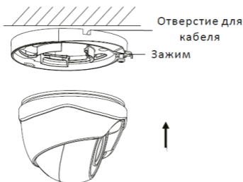
Рисунок 2-7 Установка камеры
