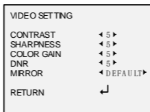
Рисунок 3-6 Настройки видео
