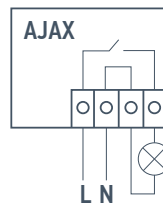
РИС. 1. Схема подключения выключателя WallSwitch
