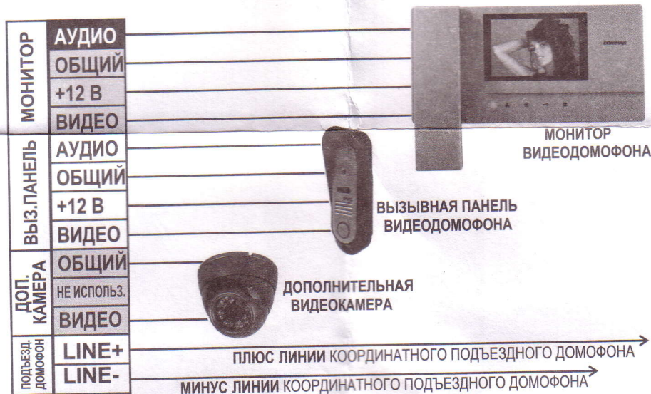
СХЕМА ПОДКЛЮЧЕНИЯ ПЛОСКОГО КАБЕЛЯ
