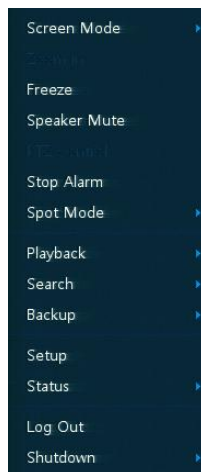
Рис. 3-4 Контекстное меню
