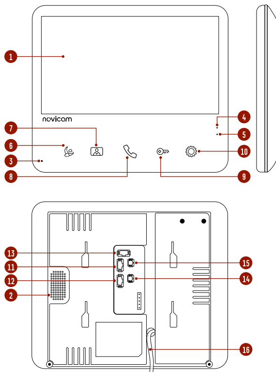
Рис. 3. Монитор видеодомофона UNIT 7
