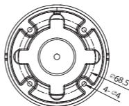
Вид снизу
