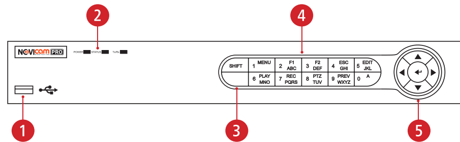
Рис. 5 Пример интерфейса передней панели TR1104F | TR1108F | TR2108F | TR2116F
