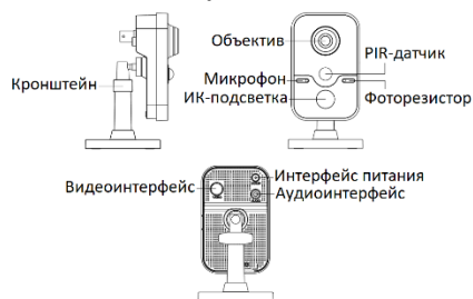
Рисунок 1-24 Компактная камера
