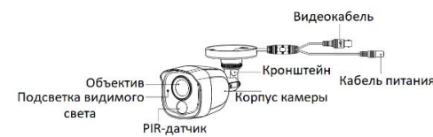
Рисунок 1-5 Цилиндрическая камера IV типа
