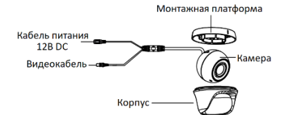
Рисунок 1-14 Камера «шар» I типа
