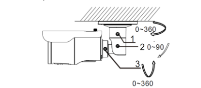
Рисунок 1-7 Настройка угла наблюдения камеры
