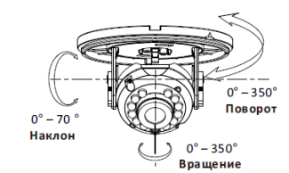
Рисунок 1-11 Настройка угла наблюдения камеры
