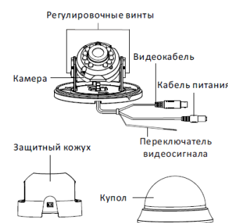
Рисунок 1-10 Купольная камера I типа
