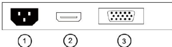
Рисунок 2-1 Интерфейсы устройства
