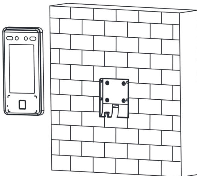
Рисунок 3-9. Установка устройства
