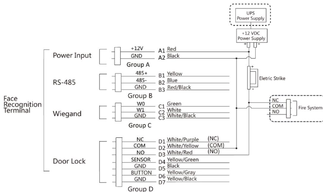
Рисунок 4-7. Подключение устройства
