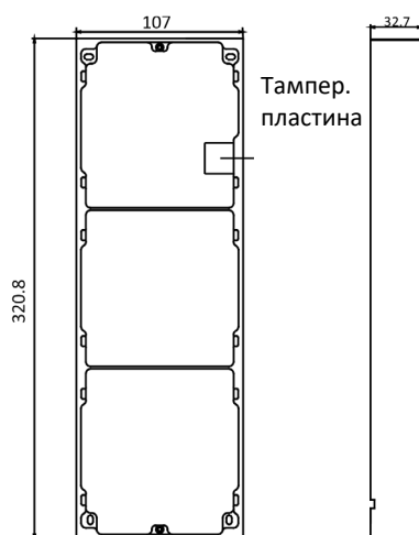
Рисунок 3-44 Монтажная рама
