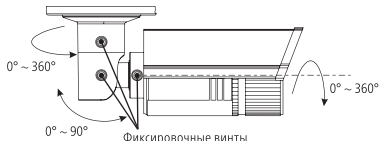
Рис. 6 Регулировка угла обзора камеры FC19W|FC29W|FC59WX
