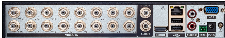
Рис. 5. Задняя панель. Внешний вид для FR1116LX
