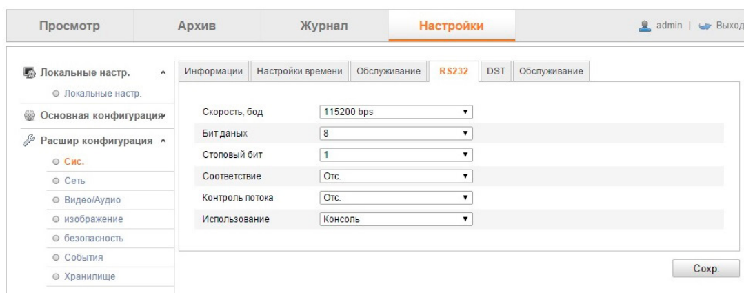
Рисунок 14. RS232/485.
