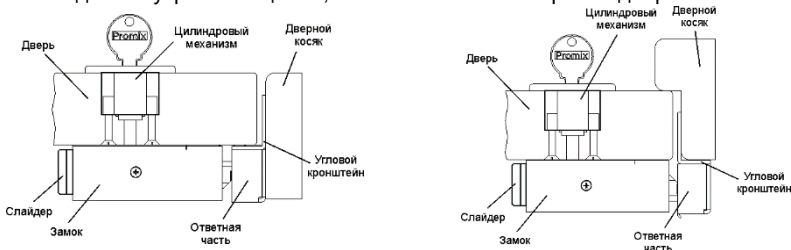
Рис. 5 – Монтаж замка на дверь открывающуюся наружу
