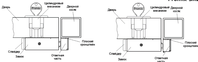
Рис. 6 – Монтаж замка на дверь открывающуюся внутрь
