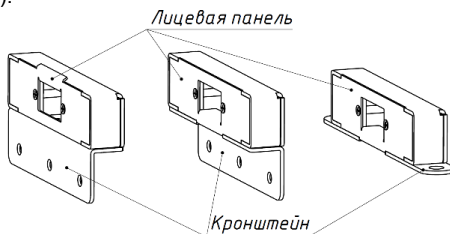
Рис. 4 – Возможные варианты сборки ответной части (внутренний/наружный варианты ответной части, вариант ответной части с плоским кронштейном)
