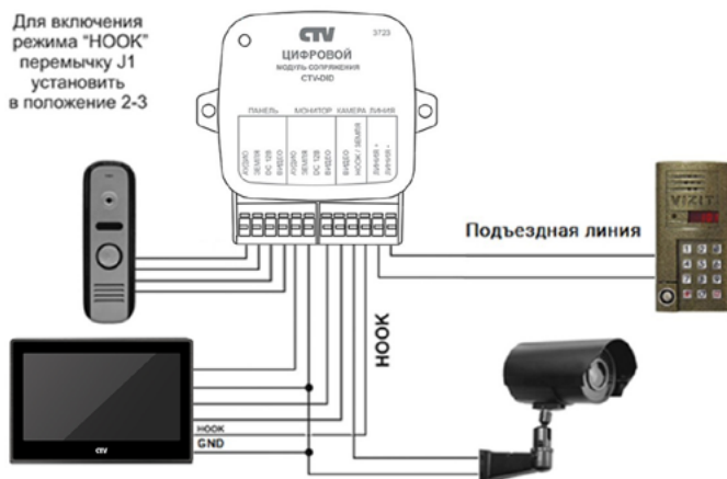
Рисунок 5 — Использование сигнала HOOK
