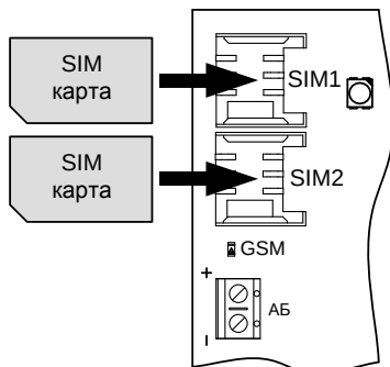
Рис.6 Установка SIM карт
