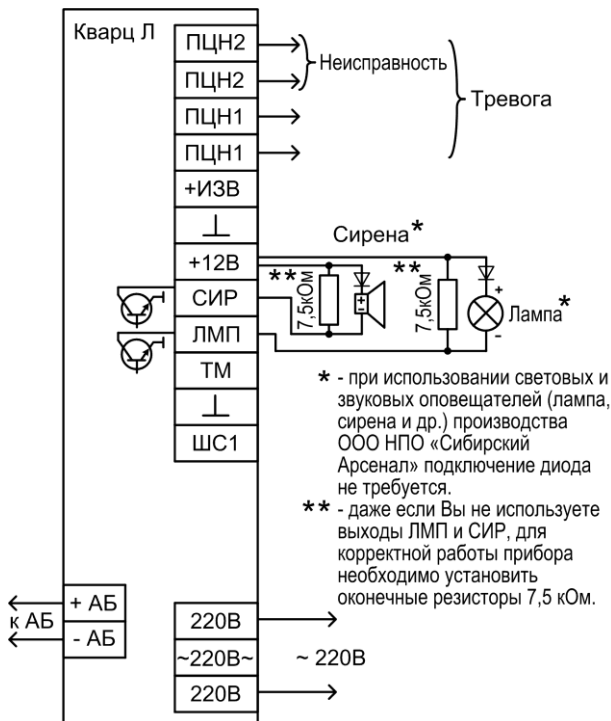
Рис.А1 Схема внешних соединений
