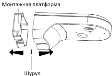
Рисунок 2-12 Демонтаж кронштейна
