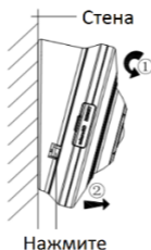
Рисунок 2-11 Демонтаж камеры
