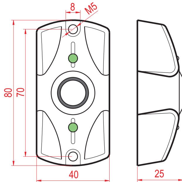
Рис. 1 Размеры
