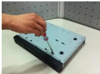
Замацуеце жорсткі дыск на ніжняй панэлі пры дапамозе шруб праз соотвѣтвующие адтуліны.
