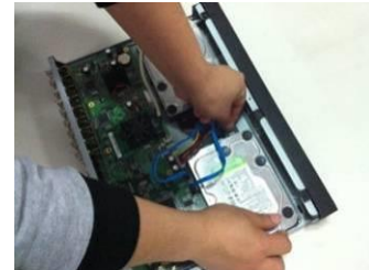
Падключыце SATA кабель і кабель харчавання на ніжняй і задняй частцы корпуса і зачыніце корпус верхняй вечкам.
